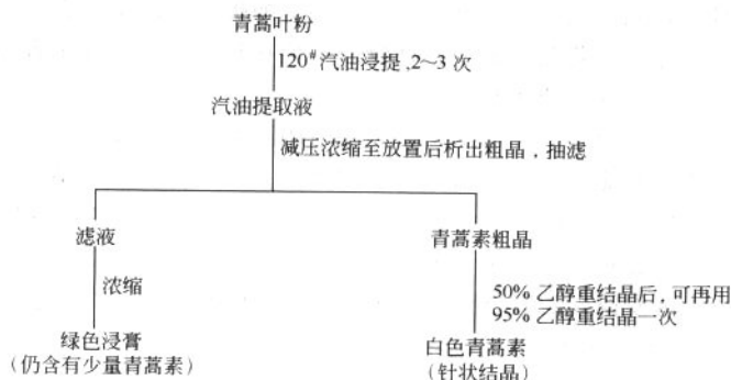
图 2-4-1 提取工艺流程简图
