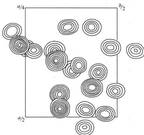
图 1-3-7 青蒿素分子沿 C 方向电子云密度叠合图
