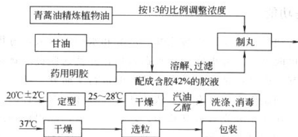
图 1-6-1 制青蒿油胶丸的工艺流程
