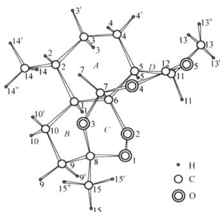
图 1-3-9 青蒿素分子的透视图
