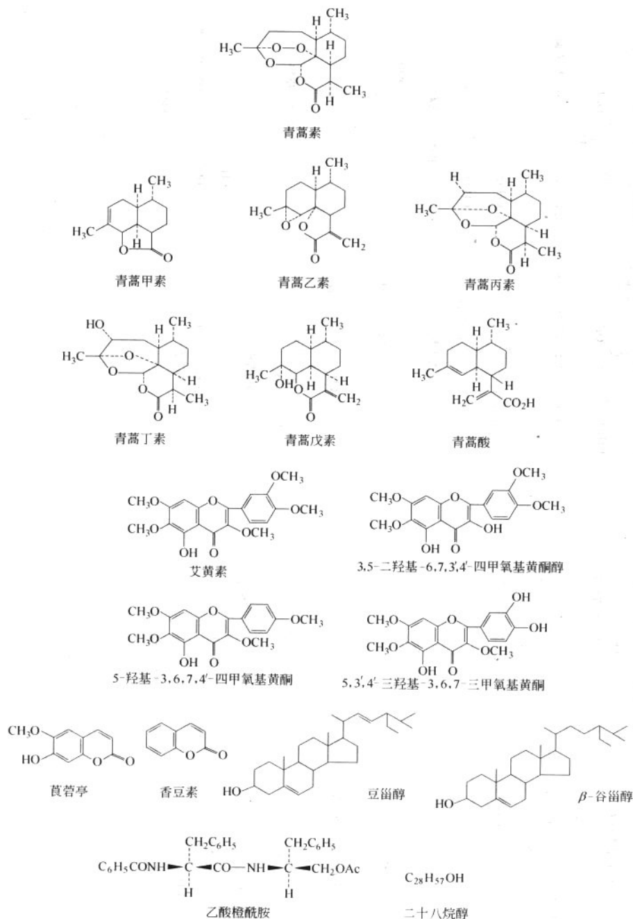
图 1-2-42 青蒿的化学成分结构式
