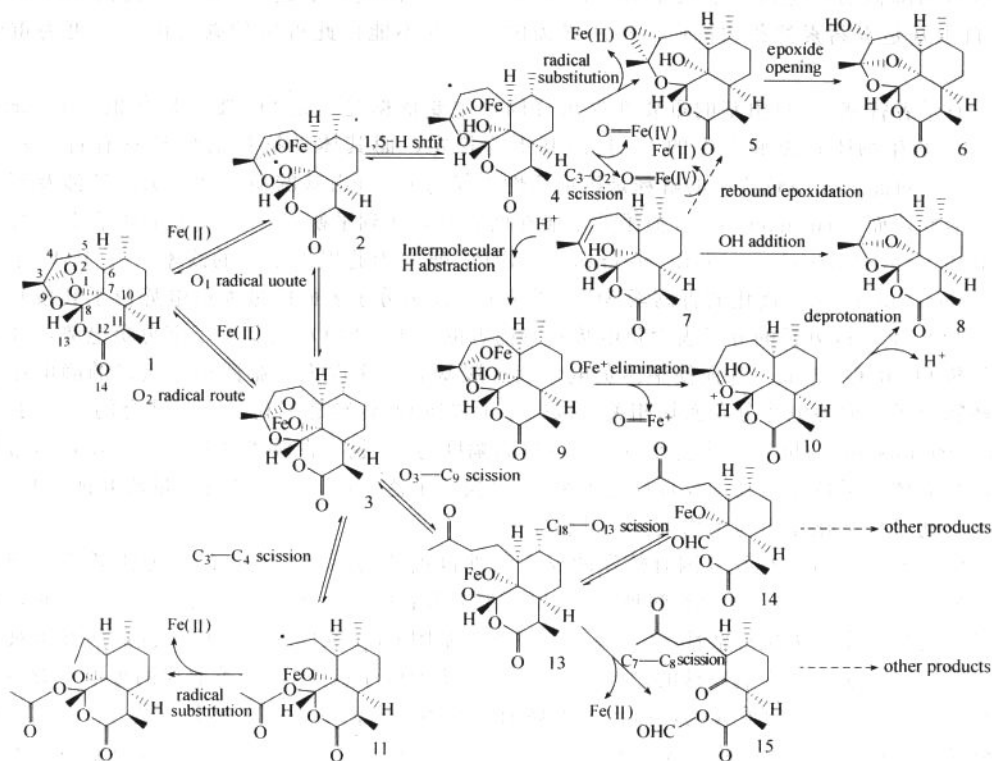
图 4-2-1 青蒿素亚铁介导下的还原裂解
