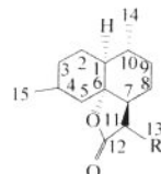
4,5 \alpha -epoxy R=CH 2
