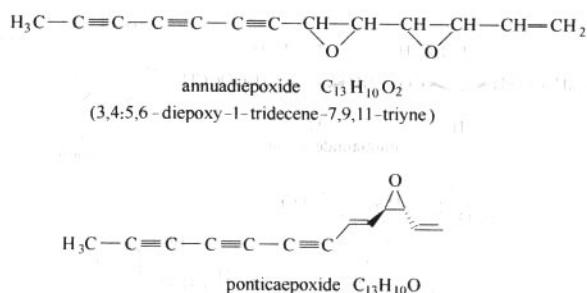
图 1-4-3 中药青蒿中分离得到的烯炔化合物结构示意图
