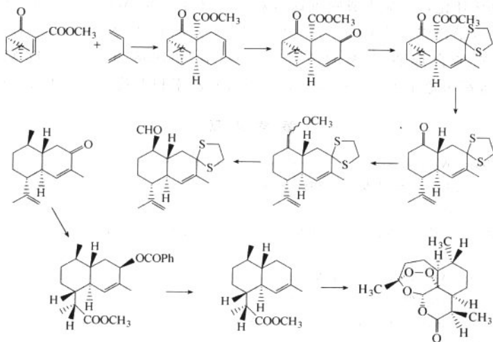
图 2-5-5 Liu's 合成路线
