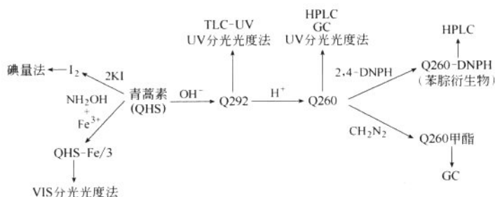
图 2-3-2 青蒿素定量反应与测定方法示意图
