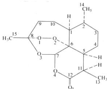
图 1-3-5 青蒿素的绝对构型
