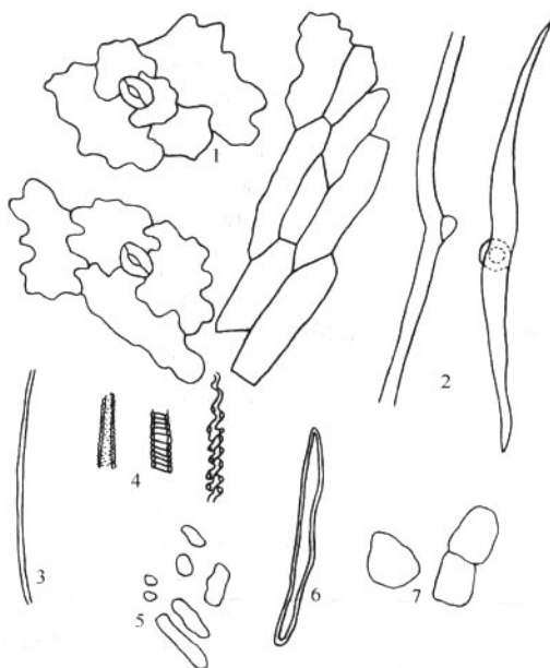
图 1-2-39 牡蒿叶粉末 (×260)
