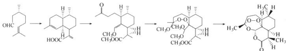
图 2-5-2 许杏祥合成路线
