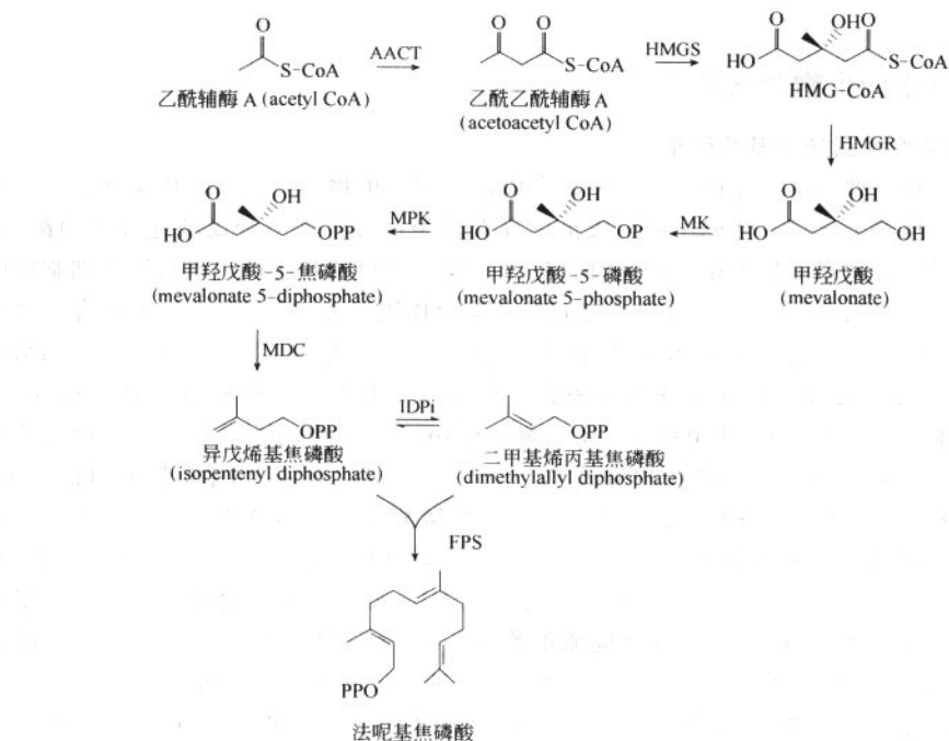
图 1-7-1 类异戊二烯甲羟戊酸途径
