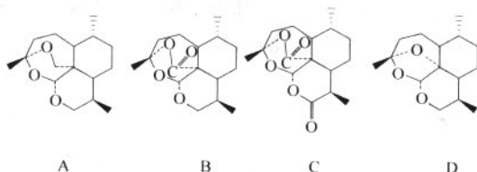
图 4-3-9 脱氧桥青蒿素结构相关化合物结构示意图
