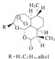
图 4-3-8 青蒿素 C 4 衍生物结构示意图
