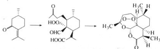
图 2-5-4 Avery's 合成路线 II
