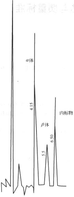
图 3-3-1 色谱图
