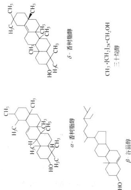
图 1-2-44 南牡蒿的化学成分结构式
