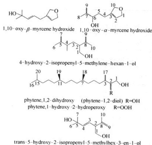
图 1-4-2 中药青蒿中分离得到的单萜与二萜类化合物结构示意图
