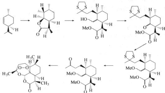
图 2-5-6 Yadav's 合成路线
