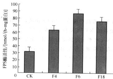
图 1-7-19 转基因青蒿的 FPS 酶活性分析
