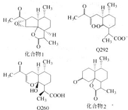
图 2-2-4 部分青蒿素酸碱反应产物结构示意图
