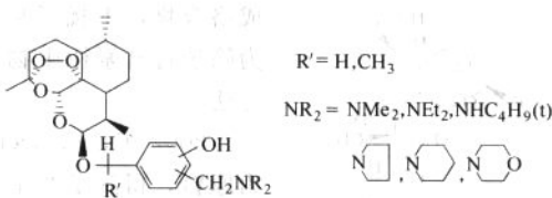
图 4-3-4 青蒿素 C 12 醚类衍生物结构示意图 III
