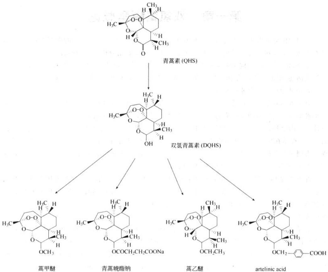
图 3-1-1 青蒿素及其主要衍生物
