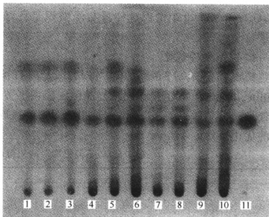
图 1-5-1 青蒿药材中青蒿素的鉴别
