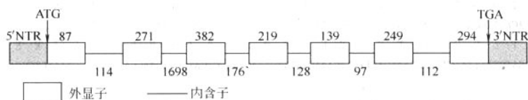
图 1-7-12 紫穗槐二烯合酶基因组 DNA 的结构
