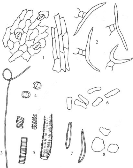
图 1-2-24 邪蒿叶粉末 (×260)
