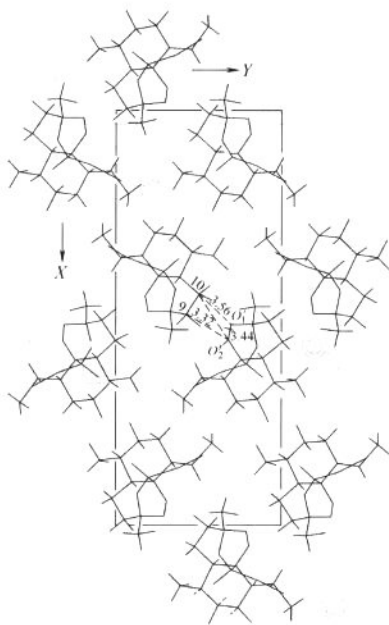
图 1-3-12 青蒿素分子在晶体中的堆积图
