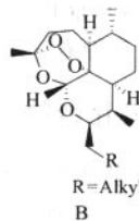
图 4-3-11 脱羰基氧青蒿素结构相关化合物结构示意图 I
