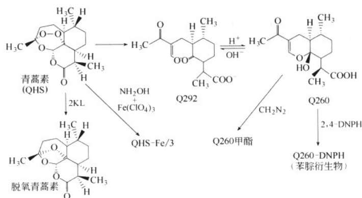
图 2-3-1 青蒿素定量反应示意图
