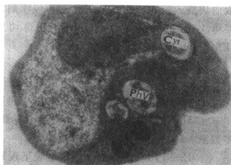
图 2-6-6 给青蒿素 (100mg/kg 组) 12h 鼠疟原虫红内期结构 ( \times 15000 ) 经口给予青蒿素, 100mg/kg, 12h, 胞口 (Cyt) 呈螺旋膜, 自噬泡 (Phv) 排出虫体
