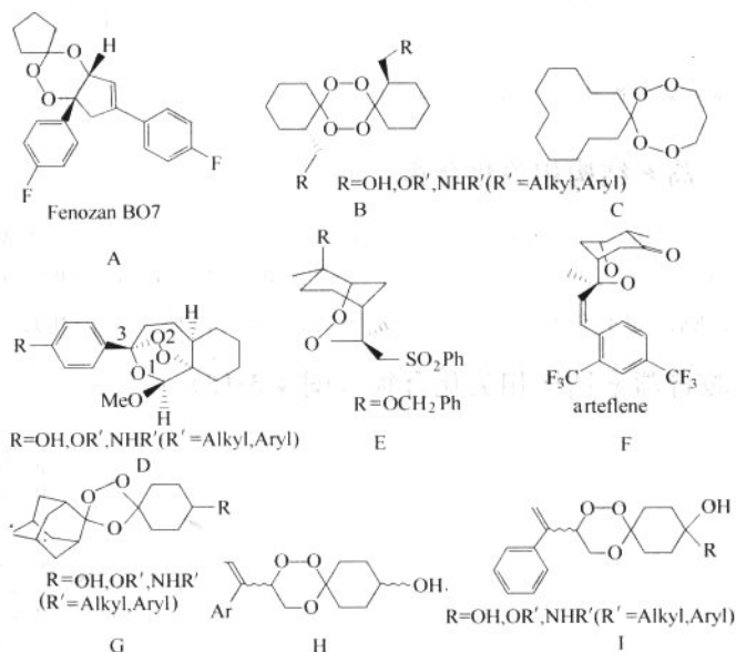
图 4-3-17 部分青蒿素结构简化物示意图
