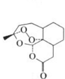
图 4-3-10 脱甲基青蒿素结构相关化合物结构示意图
