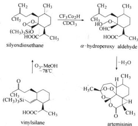
图 2-5-3 Avery's 合成路线 I
