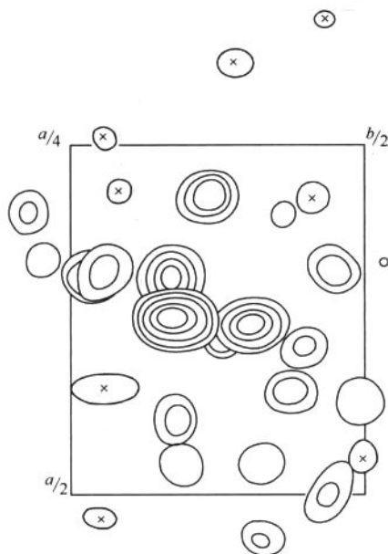
图 1-3-6 沿 C 方向的 E 图叠合图
