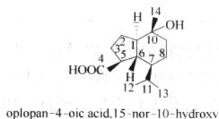
图 1-4-1 中药青蒿中分离得到的倍半萜类化合物结构示意图
