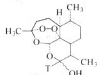
图 3-4-5 双氢青蒿素
