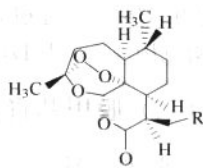
图 4-3-7 青蒿素 C 13 衍生物结构示意图
