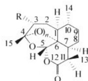
artemisinin (Qinghaosu)
