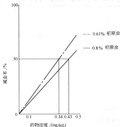
图 3-4-3 体外测定双氢青蒿素效果图
