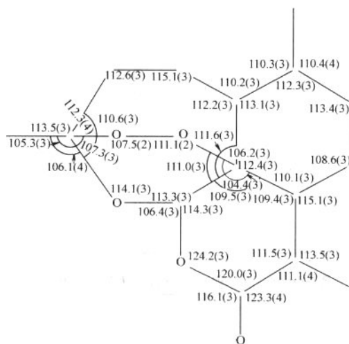
图 1-3-11 青蒿素分子中碳氧原子间键角
