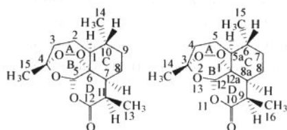
图 4-3-1 青蒿素类化合物编号示意图
