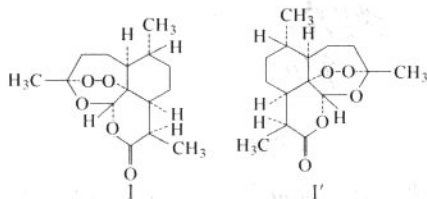
图 1-3-4 青蒿素的绝对构型
