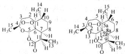
图 2-2-1 青蒿素的结构示意图
